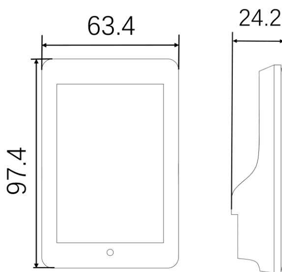
仪表主体外形
